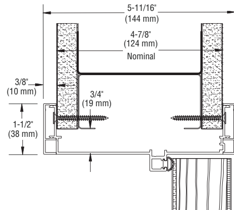
② Door Header
